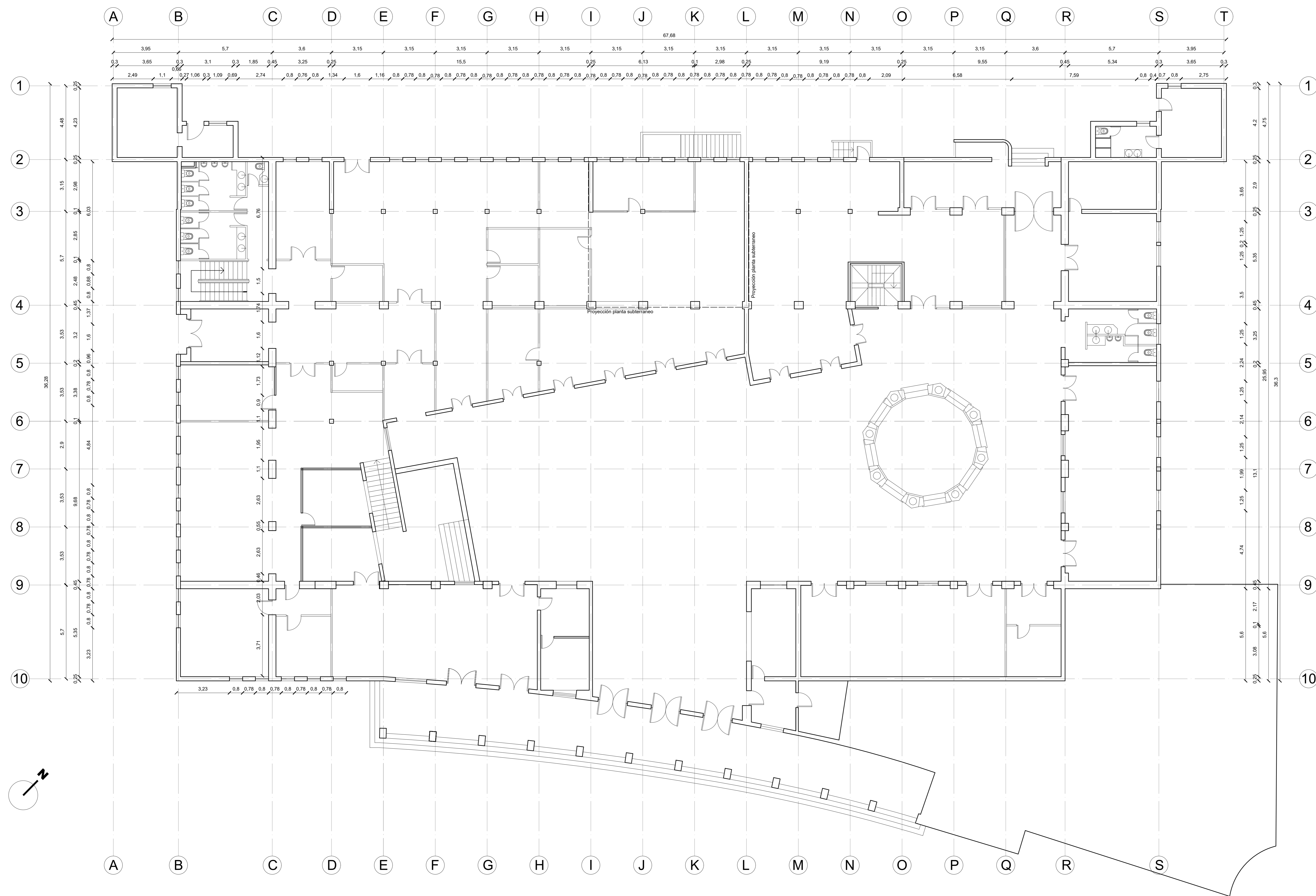
PLANTA 1° PISO Escala 1/100
